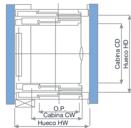
CROQUIS DE PLANTA Dos accesos puerta telescópica
